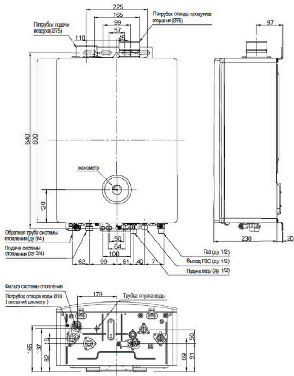
ЧЕРТЕЖ ВНЕШНЕГО ВИДА
